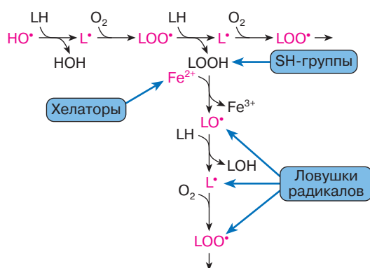
Рис. 5. Антиоксиданты, тормозящие развитие цепных реакций в липидной фазе. Цепные реакции “ведут” свободные радикалы липидов ( L\cdot и LOO\cdot ), разветвление цепей происходит при взаимодействии продукта перекиса липидов – гидроперекиси липидов ( LOOH ) с ионами Fe^{2+} . Все соединения, снижающие концентрацию перечисленных веществ, выполняют функцию антиоксидантов. Сюда относятся ферменты фосфолипаза и глутатионпероксидаза, ловушки радикалов, которые называют иногда “липидными антиоксидантами”, соединения, связывающие железо (комплексоны)
