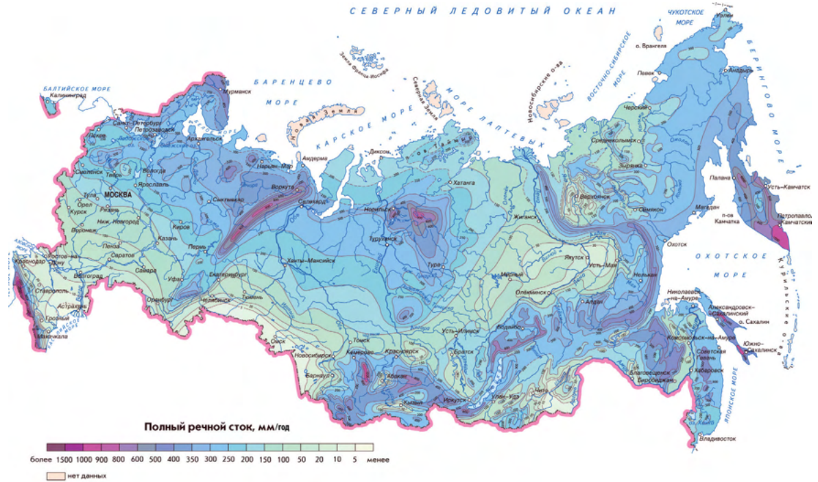
Рис. 2.14. Карта речного стока России, мм/год
