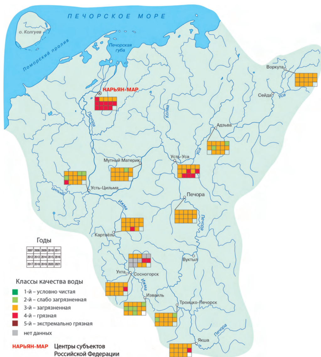
Рис. 8.5. Бассейн реки Печоры
