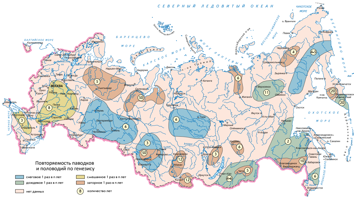
Рис. 3.16. Повторяемость паводков и половодий
