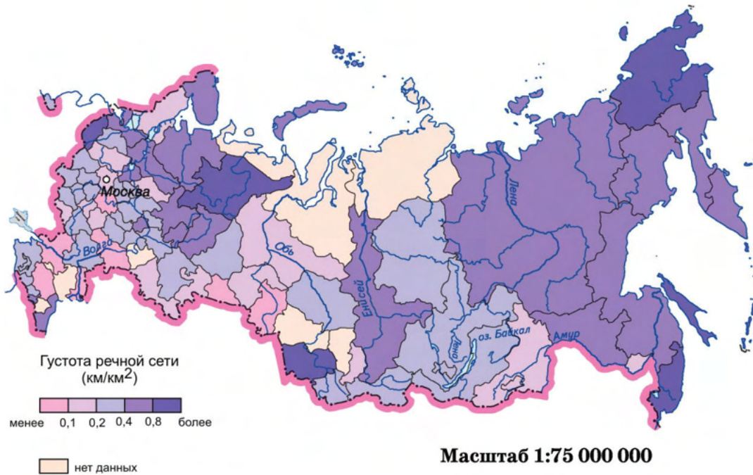
Рис. 2.13. Густота речной сети в России, км/км 2
