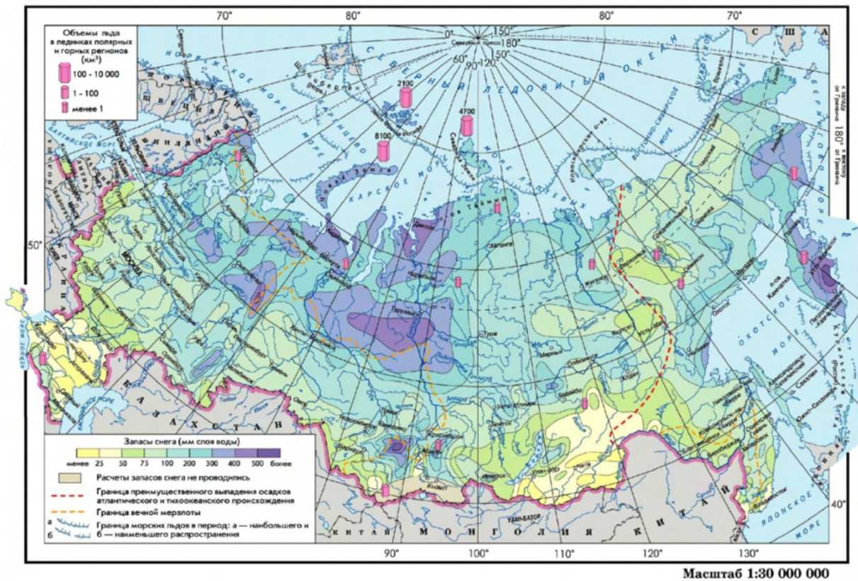
Рис. 2.47. Запасы льда в ледниках полярных и горных районов
